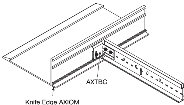
AXTBC – T-Bar Connector Clip
